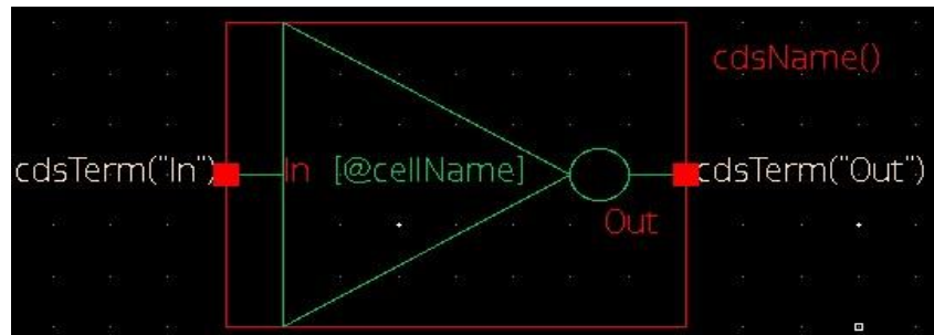
Hình 1-17: Tạo viền cho symbol inverter
