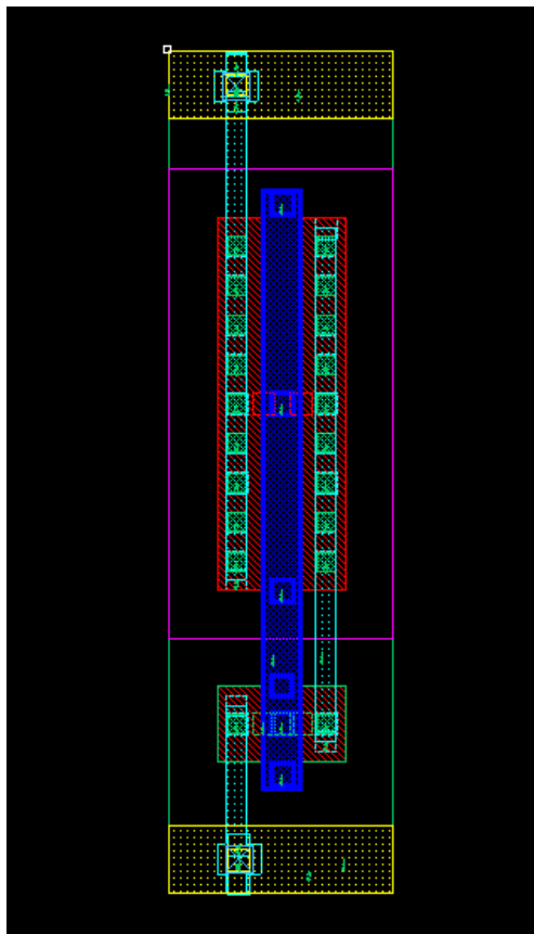
Hình 1-48: Tụ, trở ký sinh trên layout của inverter
