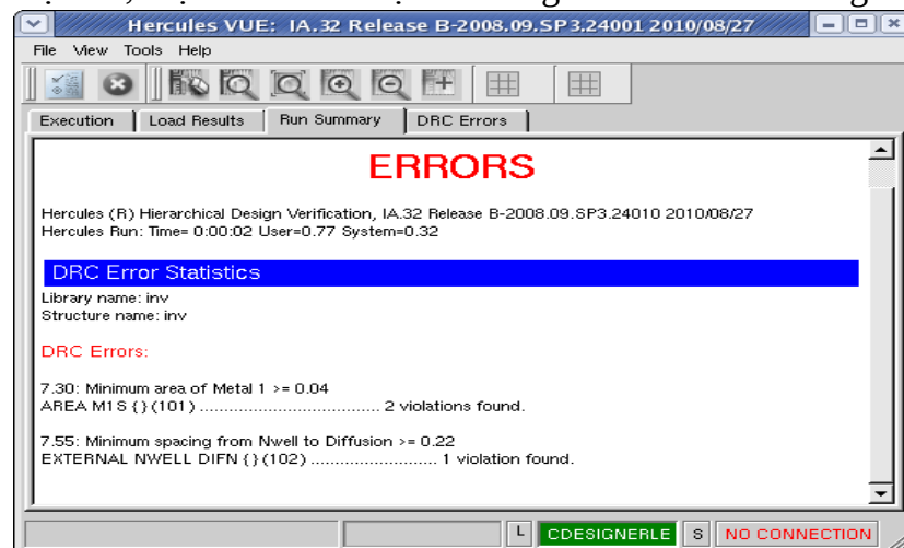
Hình 1-43: Cửa sổ thông báo lỗi DRC
