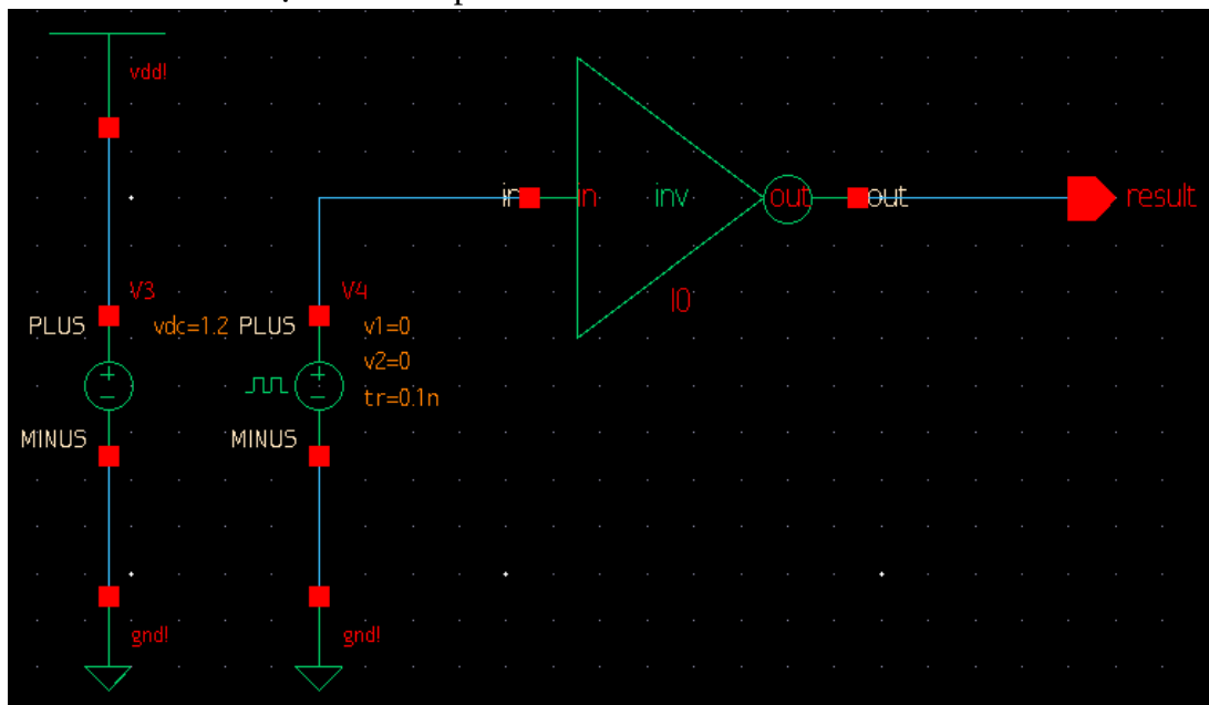
Hình 1-20: Mạch test-bench hoàn chỉnh
