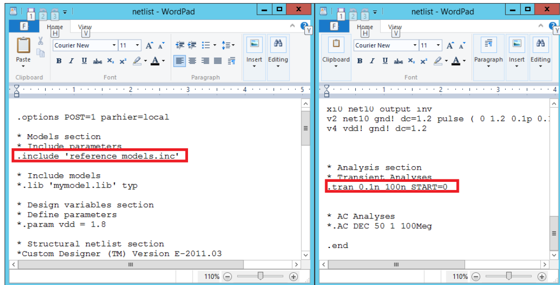
Hình 1-30: Thông số cần được chỉnh sửa
