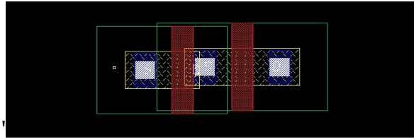
Hình 1-34: Hai CMOS khi chưa có mối nối chung Bỏ nhấn chuột, hai cực của hai CMOS tự động nối liền với nhau
