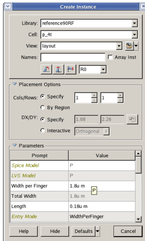
Hình 1-36: Thông số PMOS ở layout
