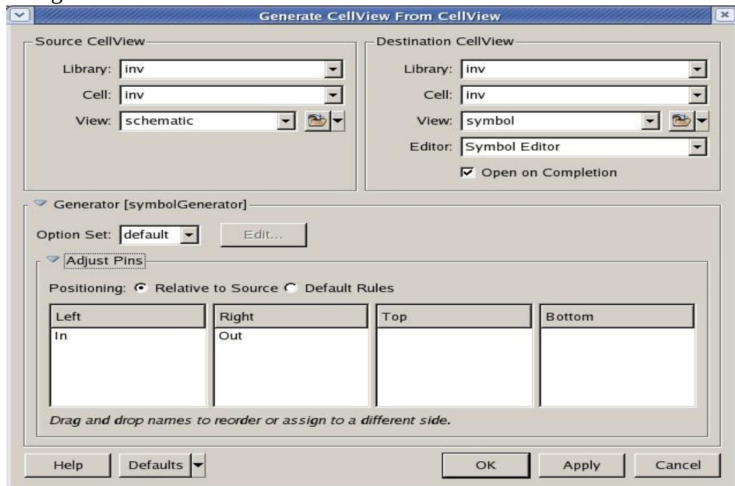
Hình 1-13: Tạo một CellView từ CellView để tạo symbol inverter Click OK → Một cửa sổ Symbol Editor hiện ra như hình dưới
