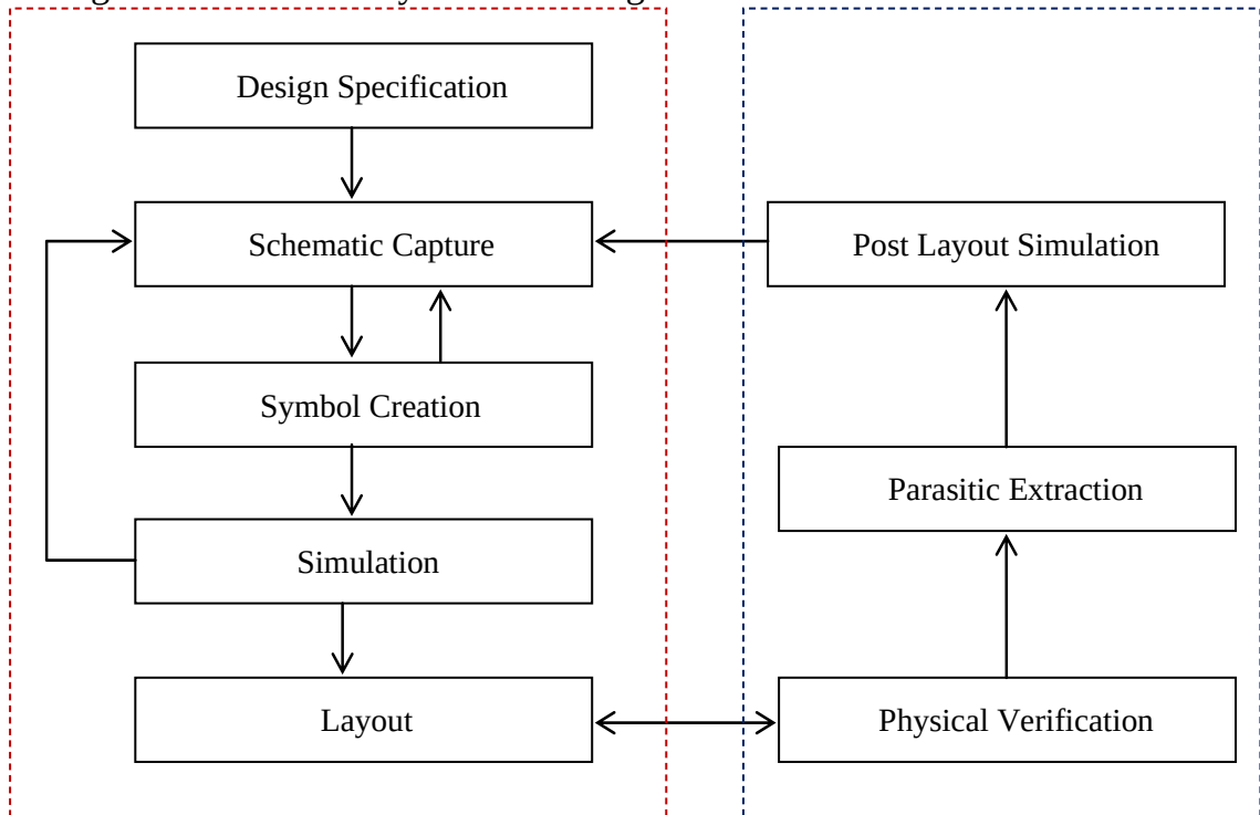
Hình 1–1: Luồng thiết kế của Custom Design
