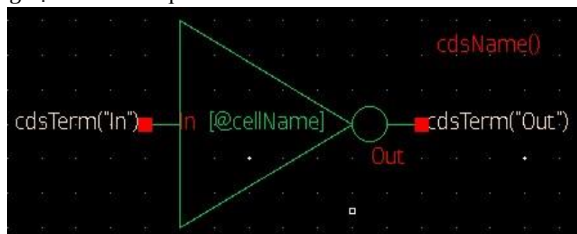
Hình 1-16: Symbol inverter
